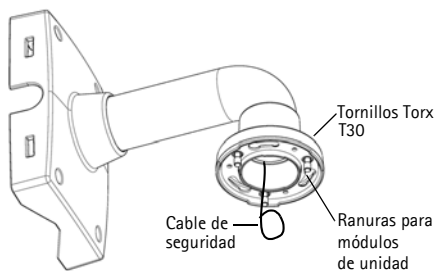
Soporte de pared (ejemplo de montaje, soporte no incluido)
