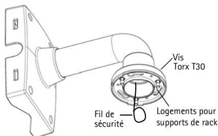
Plaquette de fixation murale (exemple de montage, plaquette non incluse)
